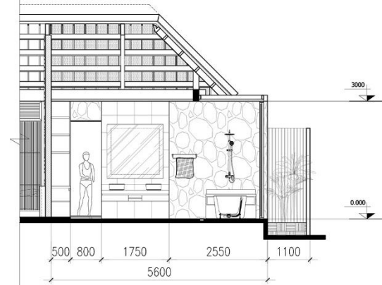
MẶT CẮT 2-2
