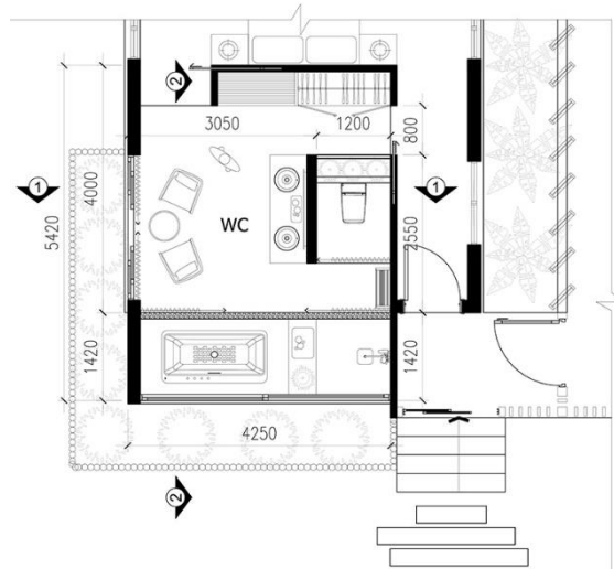
MẶT BẰNG TRÍCH ĐOẠN PHÒNG TẮM
