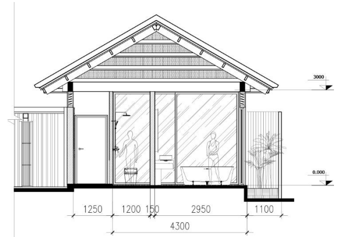
MẶT CẮT 1-1
