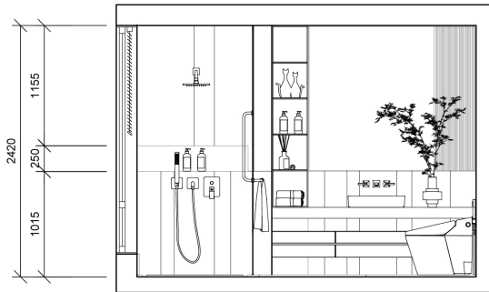
Elevation BB
